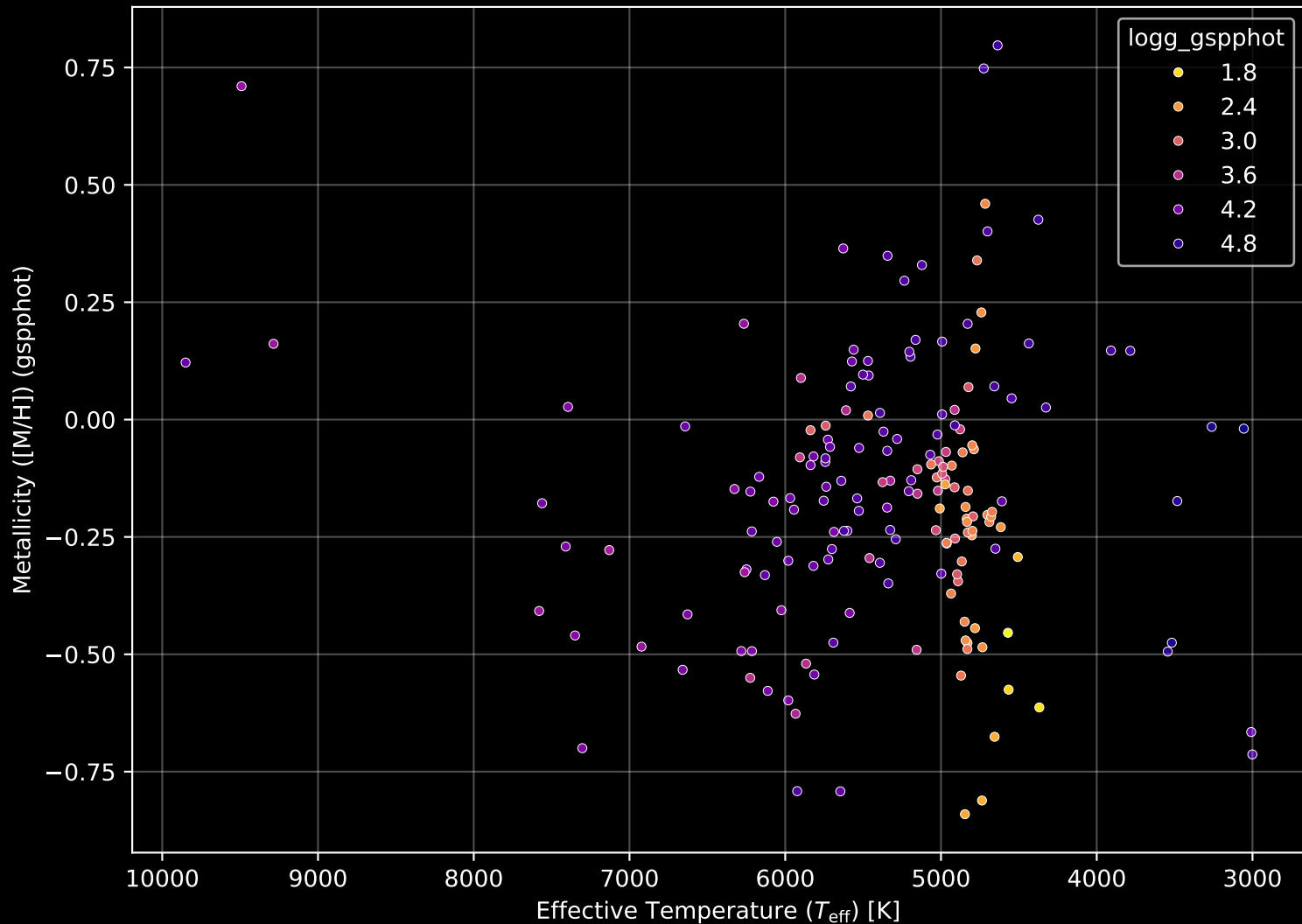
APOGEE DR17 Field: [CVZTILE_093+37_btx] Stellar Population Parameters (n= 177)
